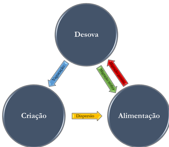
Figura 34 - Circuito migratório das lagostas.
