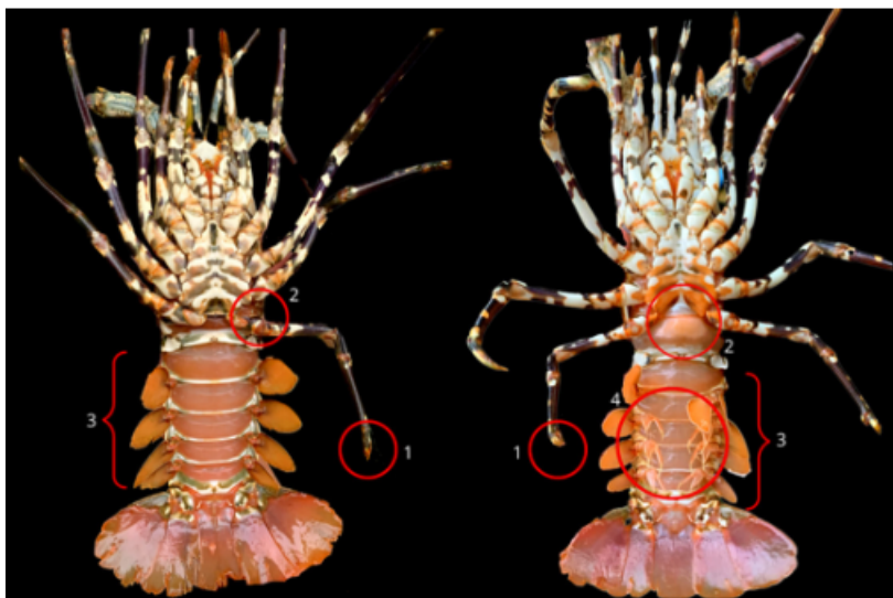
Figura 28 - Dimorfismo sexual entre lagostas machos e fêmeas. Macho à esquerda: (1) pontas pontiagudas do quinto par de patas; (2) orifício genital na base do quinto par de patas; (3) pleópodos únicos. Fêmea à direita: (1) ponta com quela no quinto par de patas; (2) orifício genital na base do terceiro par de patas; (3) pleópodos duplos; (4) pleópodos usados para segurar os ovos.
